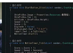
C# 着陸ゲーム
